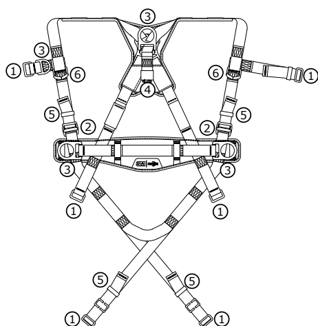
Nákres 1 – Kovové časti
