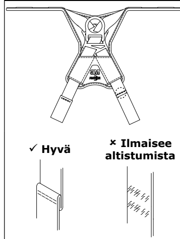
Kaavio 3 – putoamisvoimalle altistumisen ilmaisin
