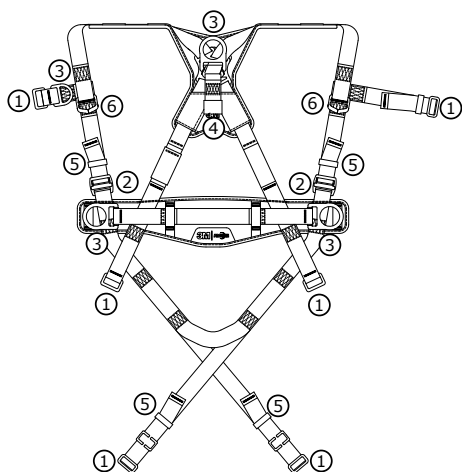
Διάγραμμα 1 – Τεχνομηχανικός Εξοπλισμός
