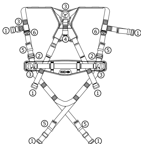
Kaavio 1 – kovat osat
