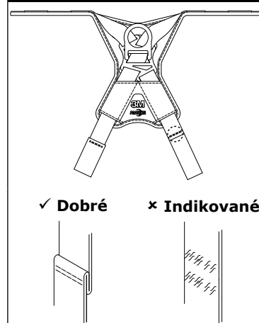
Nákres 3 – Indikátor nárazu
