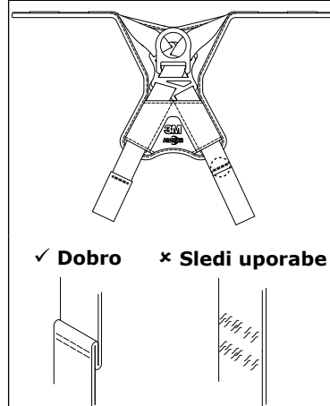
Diagram 3 – Indikator udarcev
