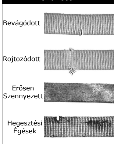
2. ábra – Heveder szövetek
