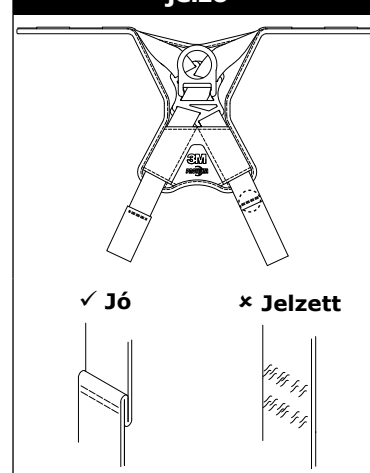
3. ábra – Zuhanásgátlás-jelző
