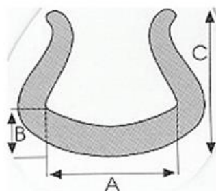
Profil U
