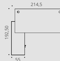
Bureau droit sur console B-box vue de dessus
