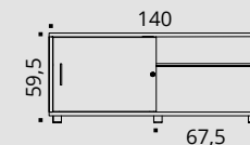
Console B-box 1 porte coulissante vue de face
