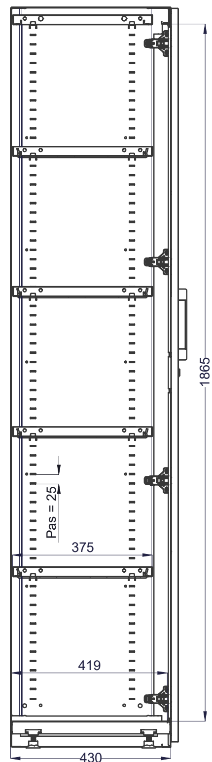
COUPE A-A
