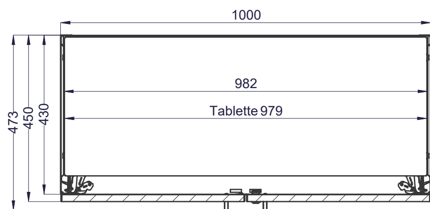
COUPE B-B
