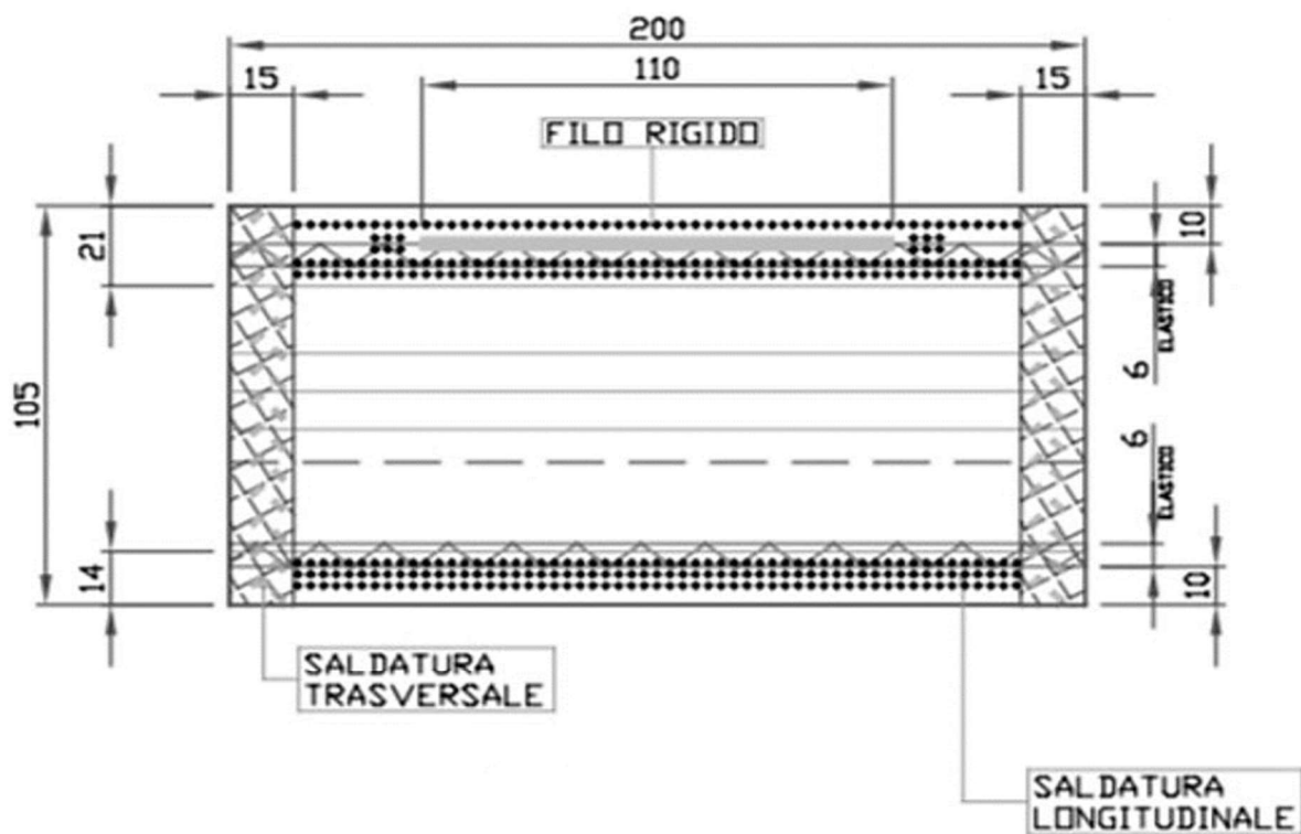
Figura 1 – Disegno
