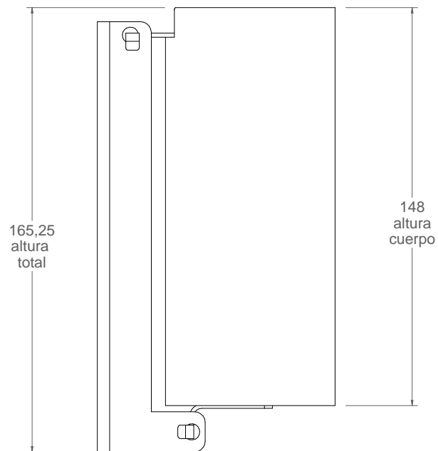
vista lateral 1:2
