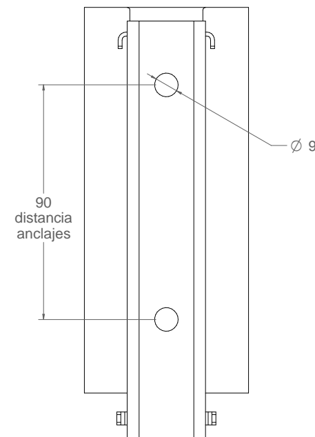
vista posterior 1:2
